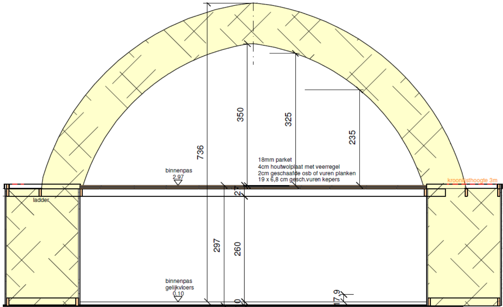
doorsnede
